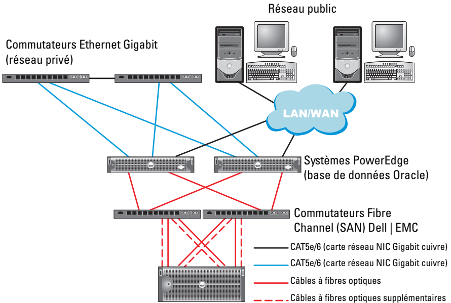
Figure 1-1. Connexions matérielles pour un cluster Fibre Channel connecté à un SAN
